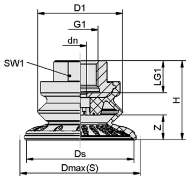
Données de construction SAB 125 HT1-60 G1/2-IG
