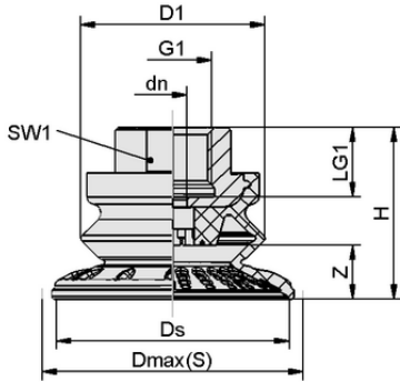
Tasarım verileri SAB 125 HT1-60 G1/2-IG
