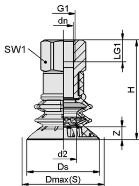
Datos de diseño SPB2f 50 SI-55 G1/2-IG
