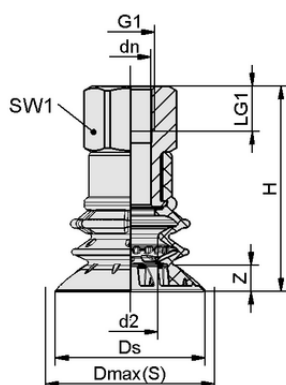
Données de construction SPB2f 50 SI-55 G3/8-IG
