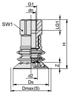
Datos de diseño SPB2f 50 SI-55 G3/8-IG
