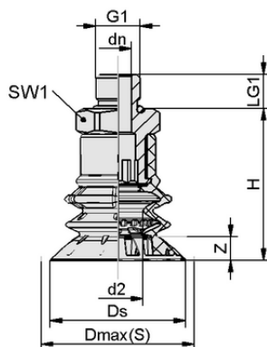
Dati di costruzione SPB2f 50 SI-55 G3/8-AG
