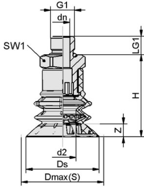
Tasarım verileri SPB2f 50 SI-55 G1/8-AG
