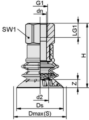
Tasarım verileri SPB2f 40 SI-55 G1/4-IG
