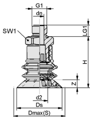
Dati di costruzione SPB2f 40 SI-55 G1/4-AG
