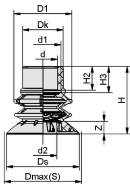
Données de construction SPB2f 30 SI-55 SC080
