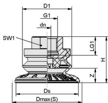
デザインデータ SAB 80 HT1-60 G1/2-IG
