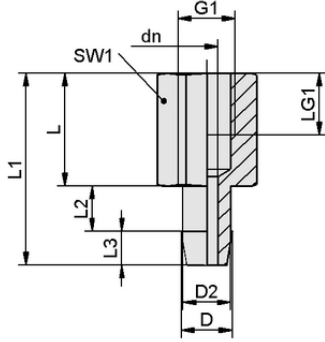
Tasarım verileri SA-NIP N057 G1/8-IG DN510
