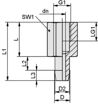
Tasarım verileri SA-NIP N056 G1/8-IG DN400
