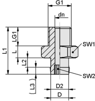
Tasarım verileri SA-NIP N056 G1/8-AG DN400
