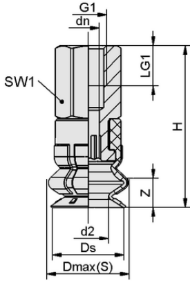
Tasarım verileri SPB1 10 ED-65 M5-IG
