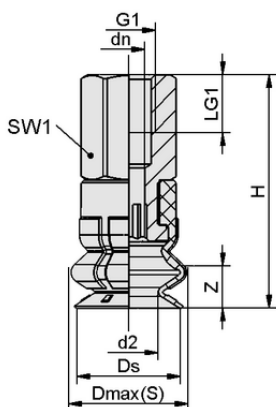
Конструктивные данные SPB1 10 ED-65 M5-IG
