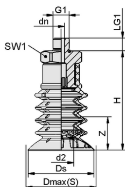
Конструктивные данные SPB4f 50 SI-55 G1/2-AG
