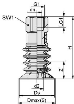
デザインデータ SPB4f 40 SI-55 G1/8-IG
