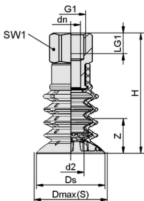
Dati di costruzione SPB4f 40 SI-55 G1/8-IG
