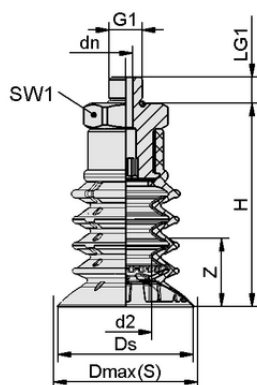
デザインデータ SPB4f 40 SI-55 G3/8-AG
