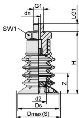
デザインデータ SPB4f 30 SI-55 G1/4-AG
