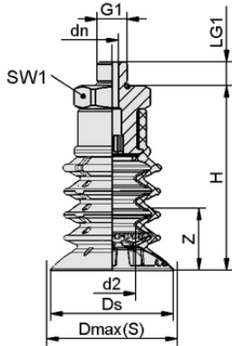
Tasarım verileri SPB4f 30 SI-55 G1/8-AG
