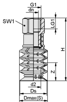
デザインデータ SPB4 50 SI-55 G3/8-IG
