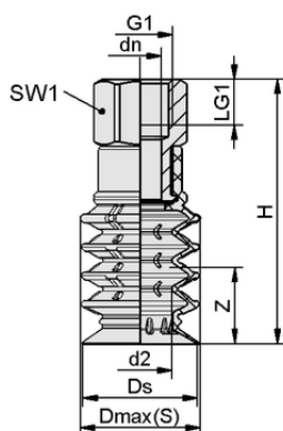
Dati di costruzione SPB4 50 SI-55 G1/4-IG
