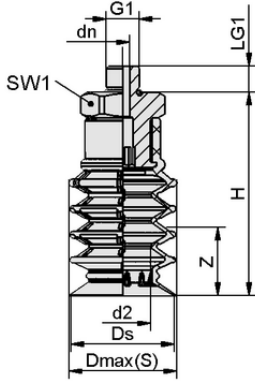
Tasarım verileri SPB4 50 SI-55 G1/2-AG
