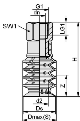
Конструктивные данные SPB4 40 SI-55 G3/8-IG
