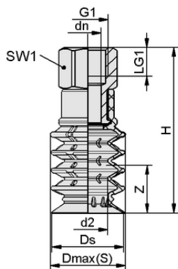
Dati di costruzione SPB4 40 SI-55 G3/8-IG
