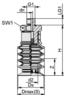
Конструктивные данные SPB4 40 SI-55 G1/2-AG
