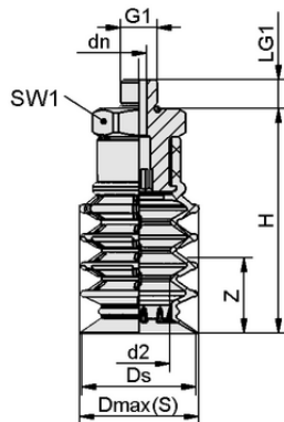
Dati di costruzione SPB4 30 SI-55 G3/8-AG
