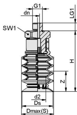
Конструктивные данные SPB4 30 SI-55 G1/8-AG
