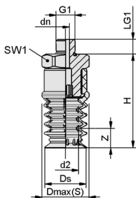
Конструктивные данные SPB4 20 SI-55 G3/8-AG
