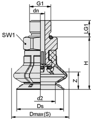
Tasarım verileri SPB1 50 ED-65 G1/4-AG
