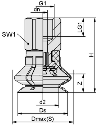
Tasarım verileri SPB1 30 ED-65 G1/8-IG
