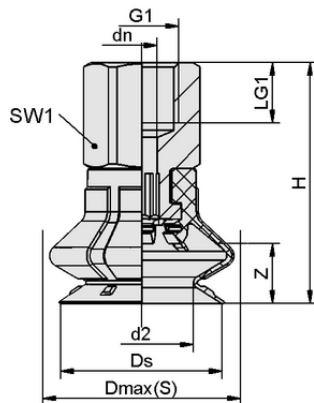
Dati di costruzione SPB1 30 ED-65 G1/8-IG
