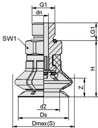
Dati di costruzione SPB1 30 ED-65 G1/8-AG
