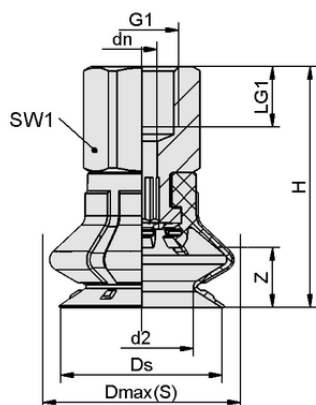
デザインデータ SPB1 20 ED-65 G1/8-IG
