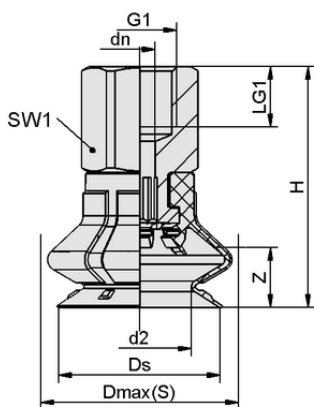
Dati di costruzione SPB1 15 ED-65 G1/8-IG
