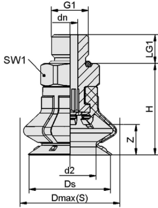
Tasarım verileri SPB1 15 ED-65 G1/8-AG
