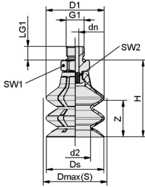
Tasarım verileri SPB2 50 ED-65 G1/4-AG
