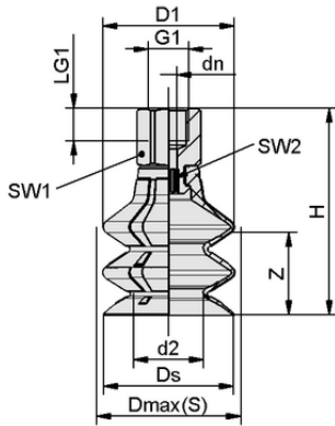
Tasarım verileri SPB2 40 ED-65 G1/4-IG
