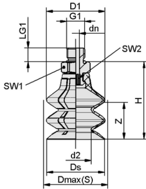
Tasarım verileri SPB2 40 ED-65 G1/4-AG
