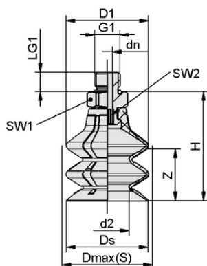
Конструктивные данные SPB2 25 ED-65 G1/8-AG
