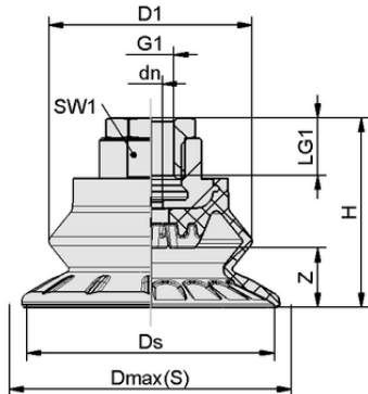
Données de construction SAB 50 HT2-65 G1/4-IG
