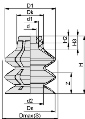
Конструктивные данные SPB2 50 ED-65 SC050
