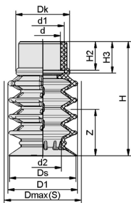
Конструктивные данные SPB4 40 SI-HD-65 SC090
