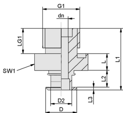
Конструктивные данные SA-NIP N043 G1/4-AG DN500
