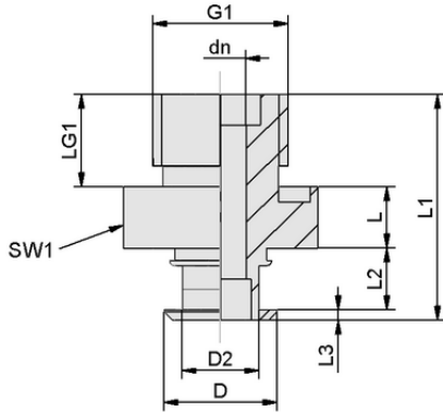
Tasarım verileri SA-NIP N043 G1/4-AG DN500
