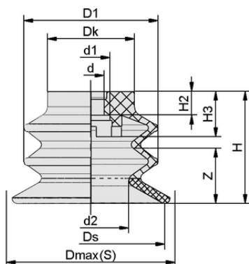
デザインデータ SDC2 50 PU 30/60 N044
