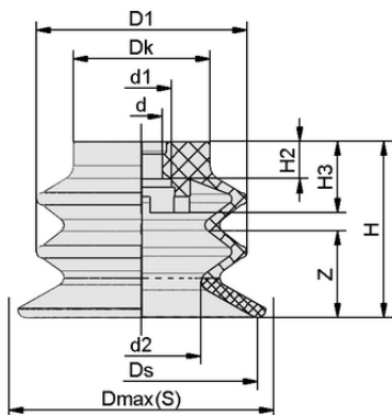
Datos de diseño SDC2 20 PU 30/60 N042
