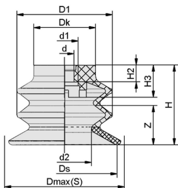
Конструктивные данные SDC2 20 PU 30/60 N042
